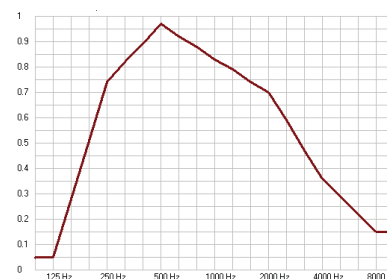
Absorption acoustique avec plenum de 40mm et laine minérale de 40mm
