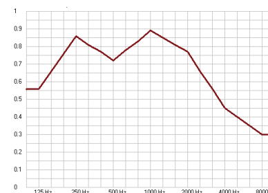
Absorption acoustique avec plenum de 200mm et laine minérale de 40mm
