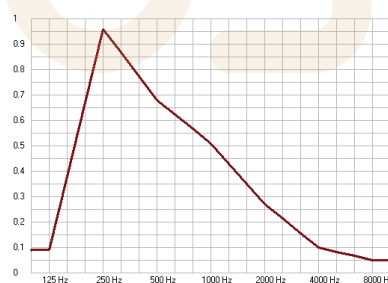
Absorption acoustique avec plenum de 40mm et laine minérale de 40mm
